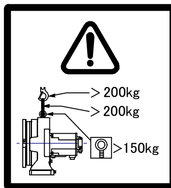
Fig. 3 (d) Transportation label
