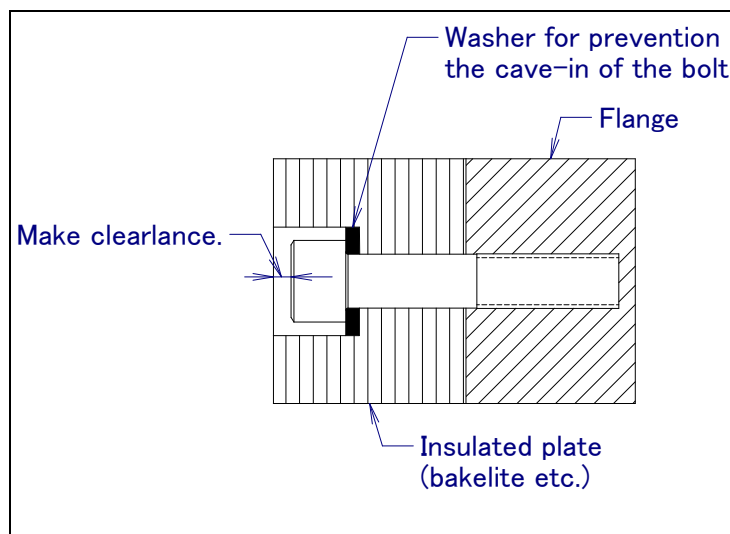
Fig. 4.1 (d) Structure for insulation
